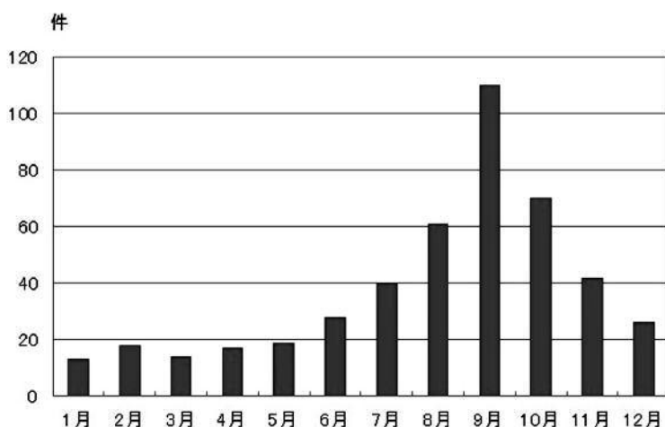
図 日本の竜巻の月別発生確認数 (1991～2017年：海上竜巻は除く)
