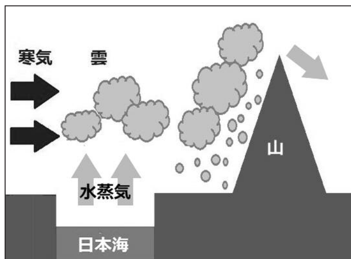
図2. 日本列島の西側に豪雪地帯が多い理由
