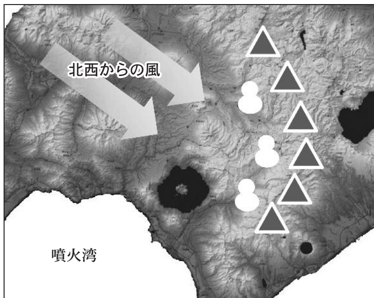
図3. 季節風の流れ込み
