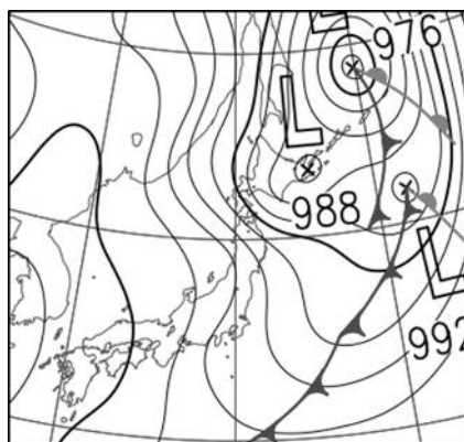
2012年11月27日9時の地上天気図 胆振地方は気圧の谷が通過し、これに伴う 着雪と暴風により送電鉄塔が倒壊した (Lは低気圧、数字の単位はヘクトパスカル)
