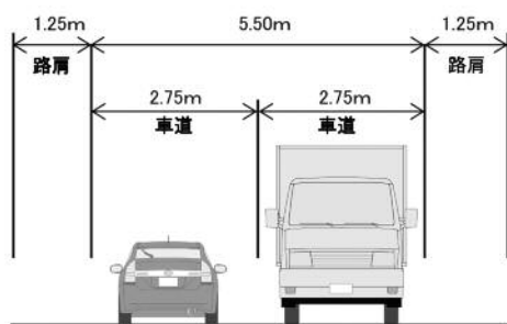
標準断面図
