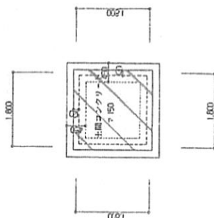
基礎伏図 1:50
